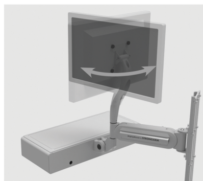
Display rotation*
